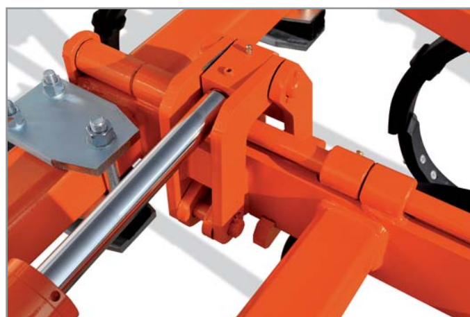
PARTICOLARE CHIUSURA IDRAULICA PARTICULAR HYDRAULIC LOCKING
